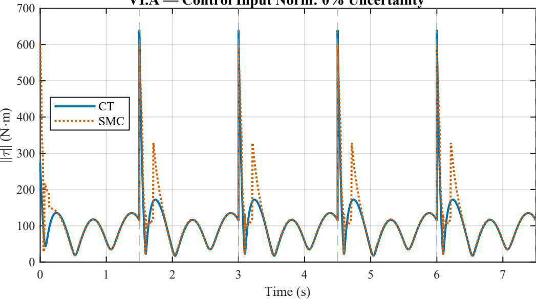
VI.A — Control Input Norm: 0% Uncertainty
